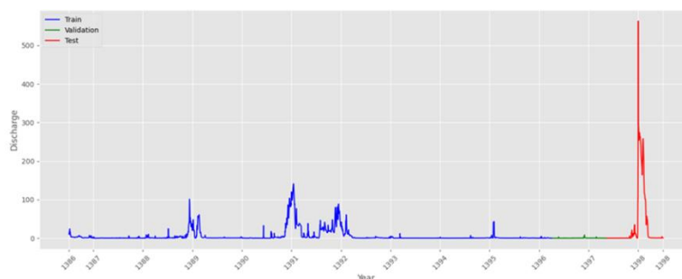
شکل ۳. داده‌های دبی ایستگاه آق‌قلا، ۱۰ سال برای آموزش، یک سال آزمایشی و یک سال جهت ارزیابی در نظر گرفته شد
